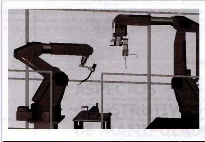
Figura 7.3 Exemplo de célula robotizada de montagem de veículos.
